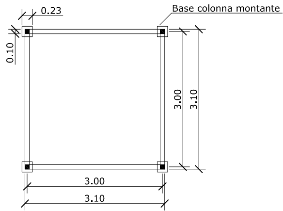
- PIANTA
