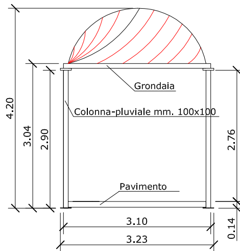
- PROSPETTO
